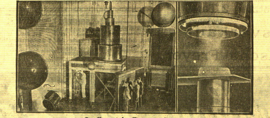
Der Apparat, der Atomgerätrümmert. In dem Hochspannungslaboratorium der A.G. in Berlin hat man mit der links abgebildeten Apparatur Spannungen von 2 1/2 Millionen Volt erzeugt, die in Verbindung mit einer von den Physikern Bräun und Lange konstruierten Röhre die Zertrümmerung von Atomen ermöglicht haben.
