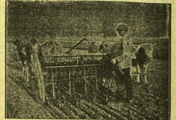
Abb. 2. Bei Verwendung der Druckrollen ruht der Samen festgebettet und keimt schneller und gleichmäßiger, ferner bleibt die Ackeroberfläche locker.
