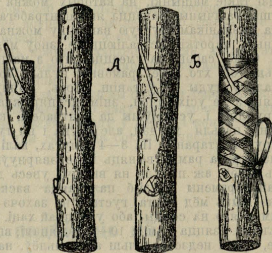
На першым рысунку з лева паказана як трэба вырэзаць ушчэпку; на другім — як трэба надрэзаць кару на дзічцы; на трэцім — як укладаць ушчэпку пад кару дзічкі і на апошнім паказана як трэба абвязываць прышчэп.
