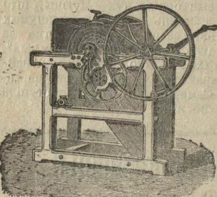
Малатарня „Kutnowianka“ штыфтовая.
