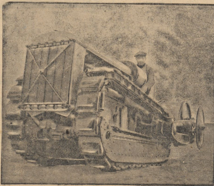
Na wystawie rolniczej w Kopenhadze ściera powszechną uwagę oryginalny plug motorowy, odznaczający się niezwykłą wszechstronnością. Plug ten może być jednocześnie użyty jako kultywator, maszyna do bronowania, wóz ciężarowy i t. d.
