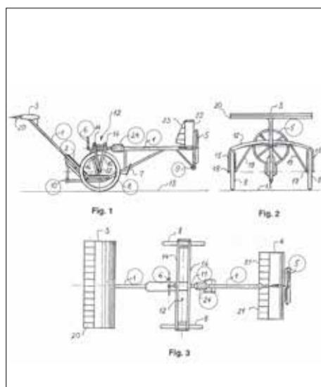
Aerodinaminis treniruoklis, patentas Nr. 6221
