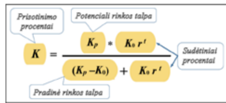
3 pav. Prisotinimo procentų (palūkanų) modelio sandara
