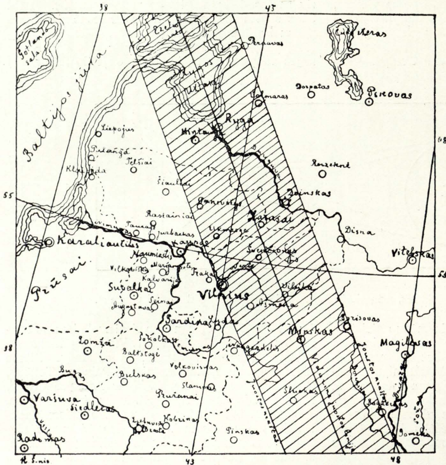
Pieš. 7. Saulės užtemimas Lietuvoje 1914 m. rugp. 821 d.
