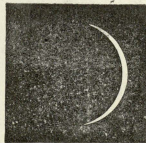
Pieš. 8. 0.95 užtemusios saulės.
