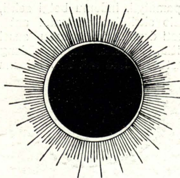
Pieš. 6. Saulės vidurio užtemimas.
