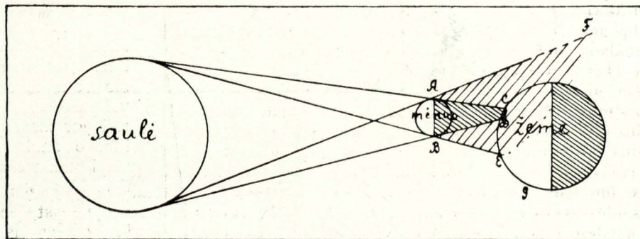
Pieš. 5. Saulės, mėnėsio ir žemės padėjimas rugp. 8 d. saulei užtemus.
