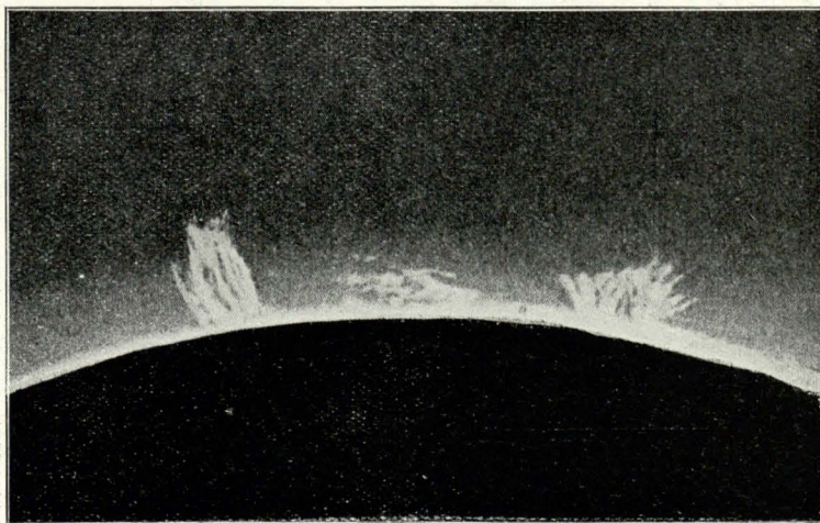
Pieš. 3. Saulės pašalys su chromosfera ir protuberansais.
