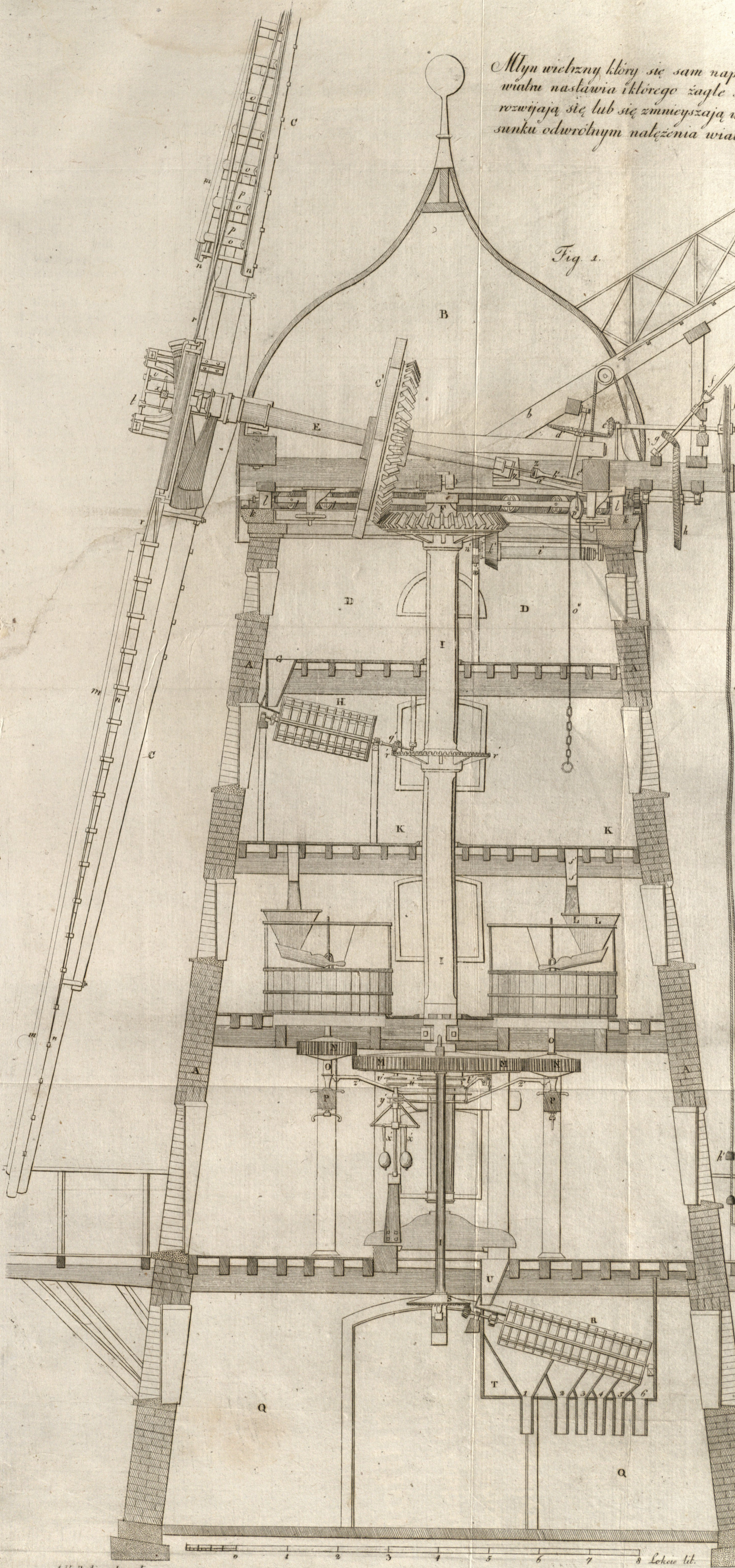
Podniesienie kamienia nieruchomego
