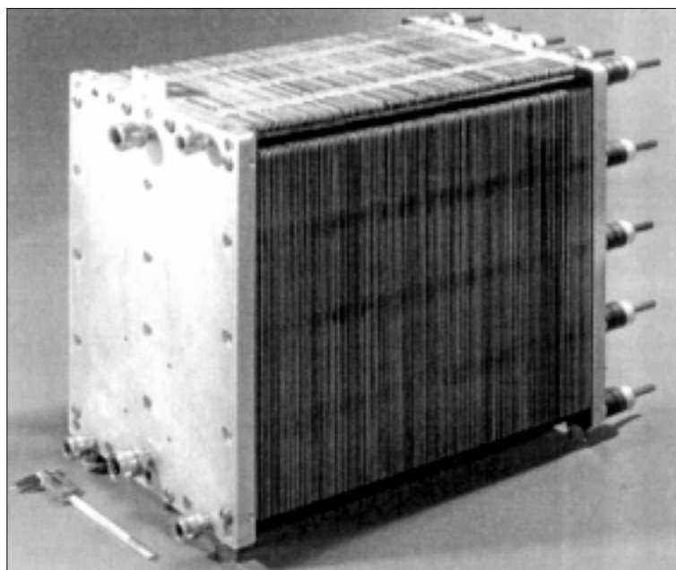
50 kW galios vandenilio jėgainės kuro elementų blokas
