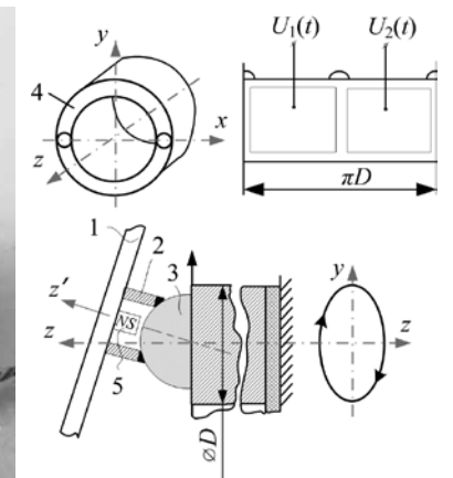
Didelės kampinės skyros lazerio spindulio deflektoriaus nuotrauka ir schema: 1 – veidrodys, 2 – pastovus cilindro formos magnetas, 3 – feromagnetinė sfera, 4 – pjezoelektrinis cilindras su sekcionuotais elektrodais
