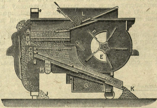
Рыс. 1. Веялка-сартыроўка.
