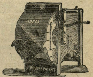
Рыс. 4. Млынок бяз сіта (сартыроўка па вазе).
