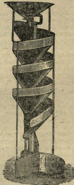
Рыс. 3. „Зьмейка“.
