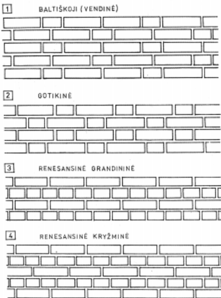
Senujų pastatų mūrų plytų perrišos būdai Lietuvoje
