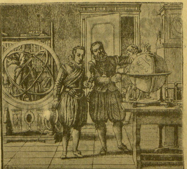
des großen Astronomen, der am 15. November 1630 starb. Durch die Entdeckung der Gesetze der Planetenbewegung wurde er der Begründer der neueren Astronomie, die sich bis zur Jetztzeit auf seine Erkenntnisse gründet. Links: Johannes Kepler mit seinem Vorkämpfer Tycho Brahe in dessen Laboratorium in Brau.
