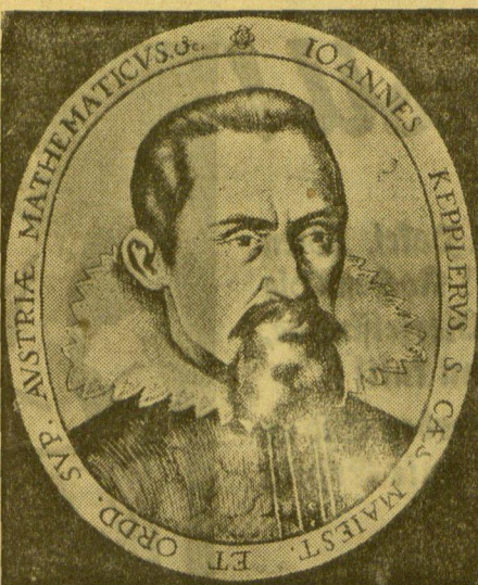
des großen Astronomen, der am 15. November 1630 starb. Durch die Entdeckung der Gesetze der Planetenbewegung wurde er der Begründer der neueren Astronomie, die sich bis zur Jetztzeit auf seine Erkenntnisse gründet. Links: Johannes Kepler mit seinem Vorkämpfer Tycho Brahe in dessen Laboratorium in Brau.
