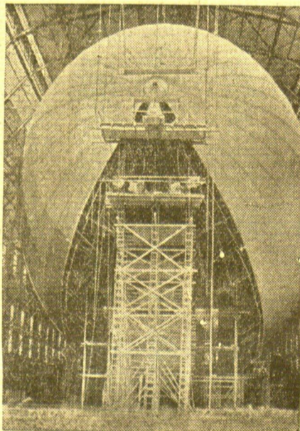
Neuester Stand der Arbeiten am „U. 130“ Blick auf die Bugspitze des im Bau befindlichen „U. 130“
