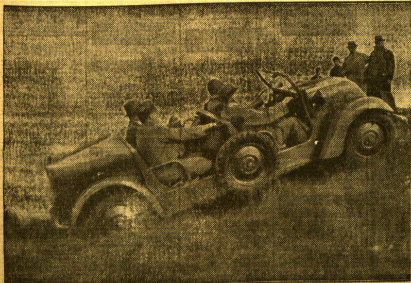
Links: Geländewagen mit Vierrad-Antrieb
