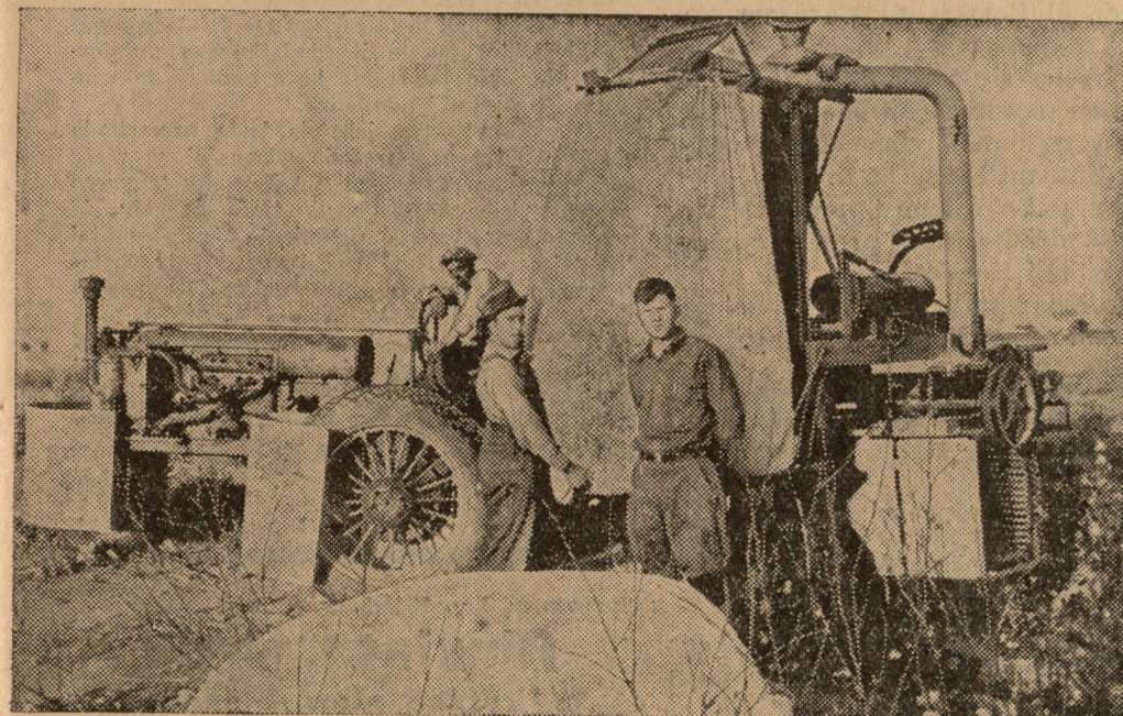
Wynaleziono maszynę do zbioru bawełny. Ze Stanów Zjednoczonych nadeszła sensacyjna wiadomość, że dwaj bracia J. D. i M. D. Rust z Memphis wynaleźli maszynę, która w ciągu godziny zbiera najmniej 1200 funtów bawełny. Dotychczas, przy ręcznej pracy, w ciągu dnia można było zbierać najwyżej 90 funtów bawełny. Jeżeli ta maszyna, którą wypróbowano już z pozytywnym wynikiem na plantacjach bawełny w Salt River Valley (stan Arizona) znalazłaby w przyszłości zastosowanie miliony ludzi, zarabiający dotychczas na kawałek chleba przy zbiorze bawełny, utraciliby pracę. Na zdjęciu maszyna z M. D. Rust na przedzie. Maszyna zbiera na walec forebki bawełny i automatycznie składa je do worka.
