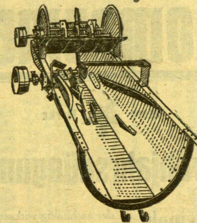
Blick in das Kopfstück der Fördermulde des Ferneinlegers mit den Aufschneidevorrichtungen
