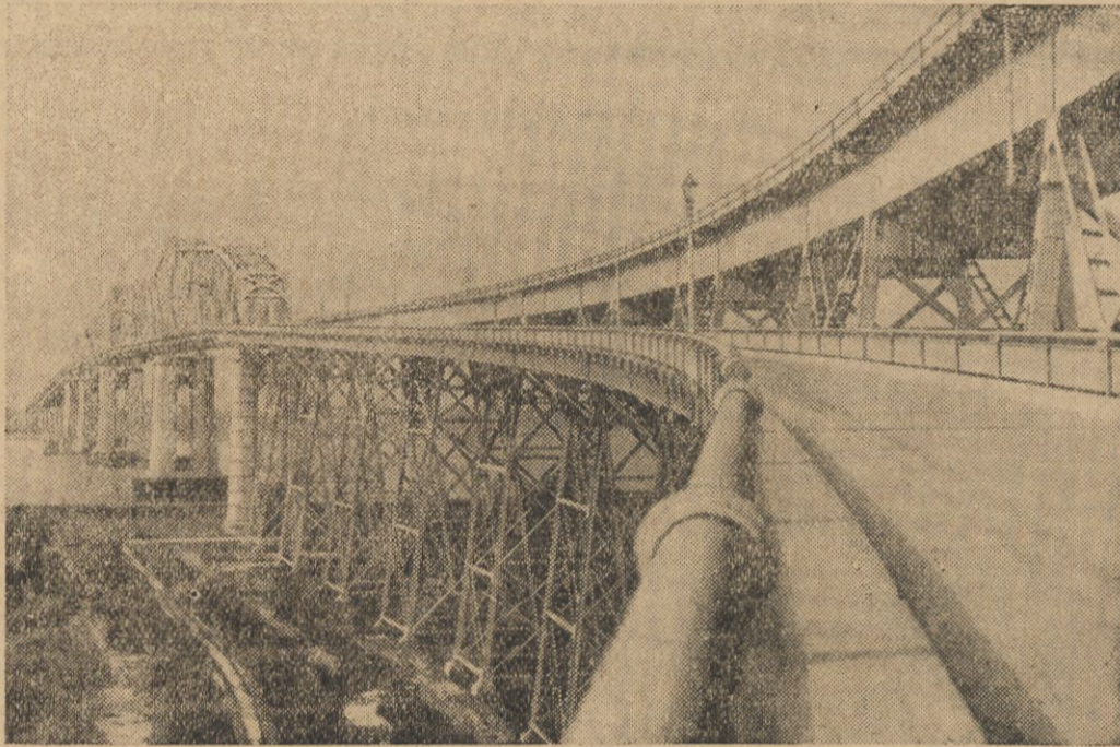
W połowie bież. miesiąca w Nowym Orleanie (stan Louisiana) odbyło się poświęcenie mostu przez Mississipi, nazwanego mostem senatora Longa ku uczczeniu jego pamięci. Most, długości 7 km., kosztował 13 milj. dolarów.
