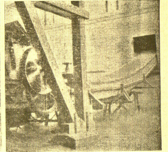
Richtig gebogene Strohschurre, die ein Herausbeulen der Ballen verhütet.
