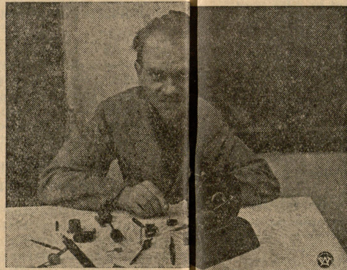
Najmniejsza na świecie maszyna. Kocis skonstruował najmniejszą na świecie maszynę parową. Waży ona 10 gramów, działa przez 10 sekund i daje 4.000 obrotów na min. Na zdjęciu — wynalazca z maszyną.
