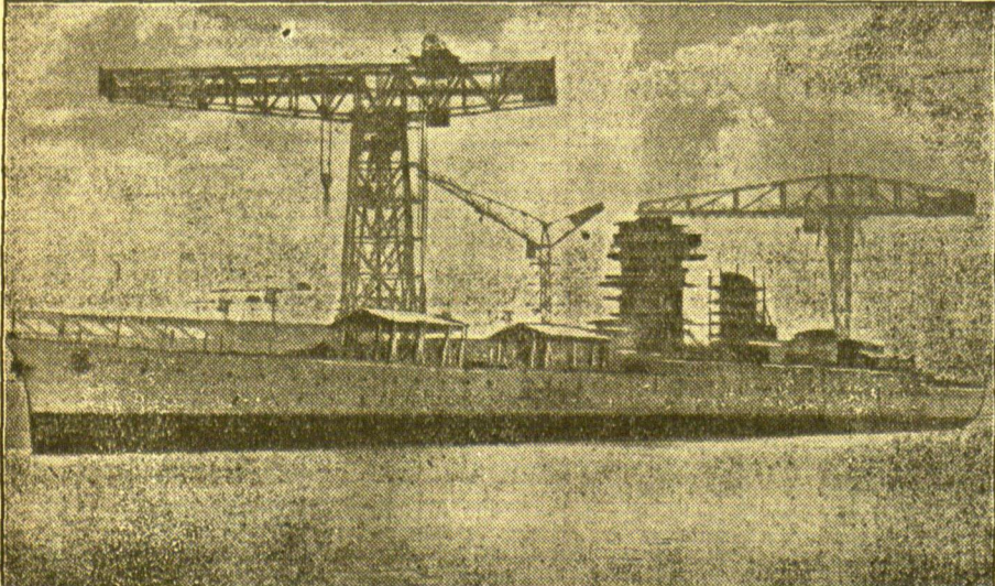
Französischer Schlachtkreuzer „Strasbourg“ vor der Vollendung Auf der Marine-Werft von Saint-Nazaire geht der neue französische 26.000-Tonnen Schlachtkreuzer „Strasbourg“ seiner Vollendung entgegen. Diese neueste Aufnahme zeigt den gegenwärtigen Stand der Bauarbeiten an dem Riesenschlachtschiff.
