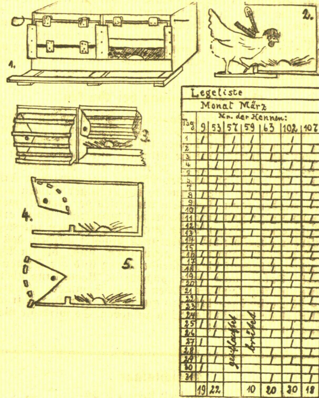
Bild 1 u. 2: Klappfallennest. Bild 3, 4 und 5: Schaukelfallennest.
