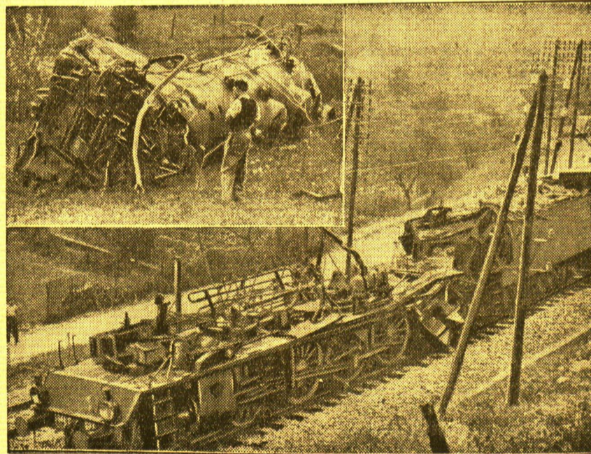
Eine Expres-Lokomotive verlor den Heizkessel während der Fahrt
