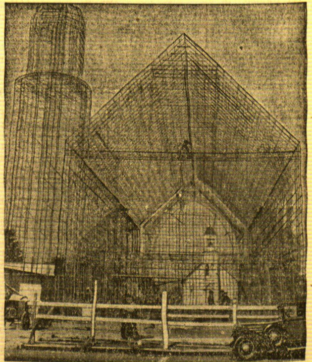
Aus diesem Stahlerüst wird eine Kirche
