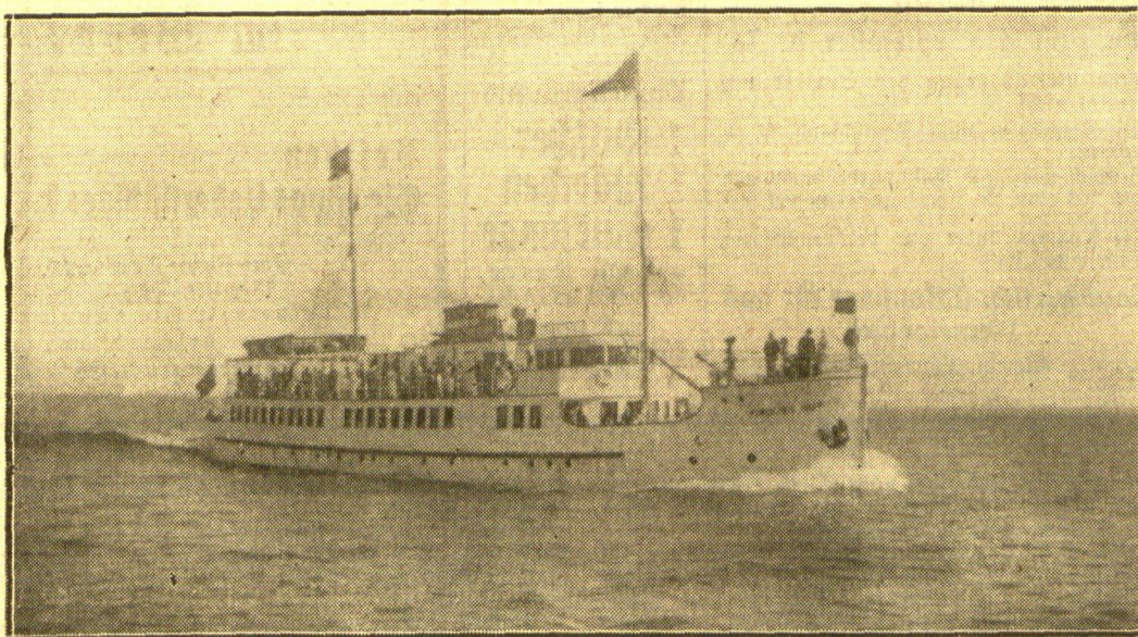
Das stolze Motorschiff „Kurisches Haff“, wie wir es alle von seinen täglichen Fahrten zu den Rehrungs- bädern kennen.
