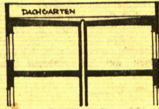
Abb. 8. Haus mit nach innen entworfenerm Flachdach durch einen Luftraum, der noch dazu beim Pfannendach durch unzählige Fugen in so enger Verbindung mit der Außenluft steht, daß bei niedriger Temperatur auch im Boden Minusgrade gemessen werden.
