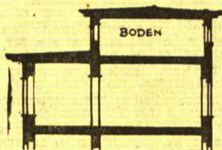
Abb. 7. Schnitt durch Obergeschloß und Boden eines Hauses mit Flachdach.
