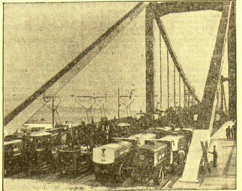
Belastungsprobe auf der neuen Wiener Reichsbrücke
