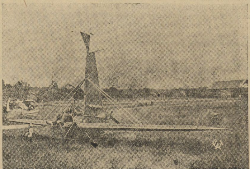
Nowy typ szybowca, zaopatrzony w motor 20-konny, nazwany przez swego wynalazcę wicehrabiego Ch. de Rogé helitrofanem. Może on lądować pod kątem 45 st. i posiada poza tem właściwości helikoptera.
