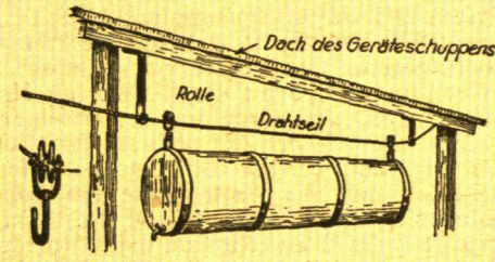
Praktische Aufbewahrung des Jauchefasses.
