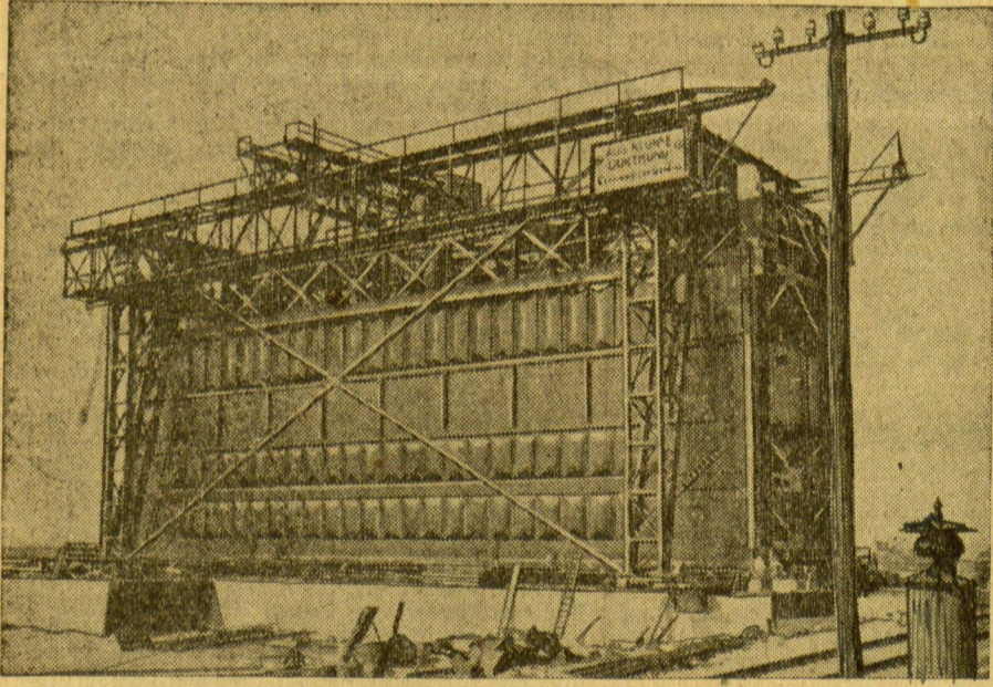
Eines der Schleuentore für Deutschlands größte Seeschleuse, die Nordschleuse in Bremerhaven, deren Bau den größten Ozeanriesen, auch der „Europa“ und der „Bremer“, das Einlaufen in den Binnenhafen ermöglichen wird. Das Schleuentor hat eine Breite von 45 Metern, während die Schleusenammer sogar 60 Meter breit und 372 Meter lang sein wird. Der Bau dieser zweitgrößten Schleuse der Welt, deren Grundstein im Frühling vorigen Jahres gelegt wurde, soll im Jahre 1932 beendet sein.
