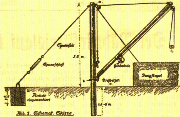
Abb. 1. Schemat. Skizze.
