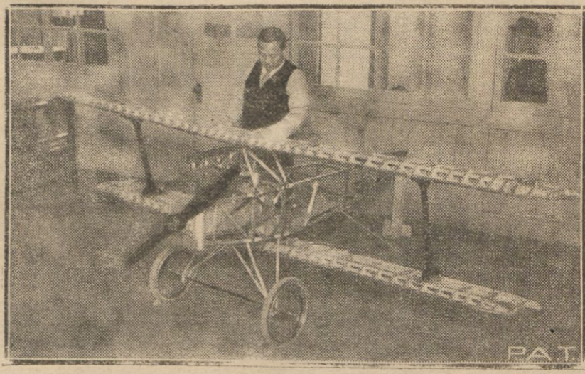
Japoński konstruktor samolotowy Okahara skonstruował nowy typ samolotu, oparty na budowie ciała ptaka, a zwłaszcza skrzydeł. Aparat ten ma mieć zapewnioną stabilizację w powietrzu dzięki specjalnemu aparatowi, który przy każdej zmianie kierunku i naporu wiatru zaczyna automatycznie działać, utrzymując aparat w równowadze i zapobiegając spadko- wi. Na zdjęciu naszym widzimy skonstruowany przez Okaharę aparat.
