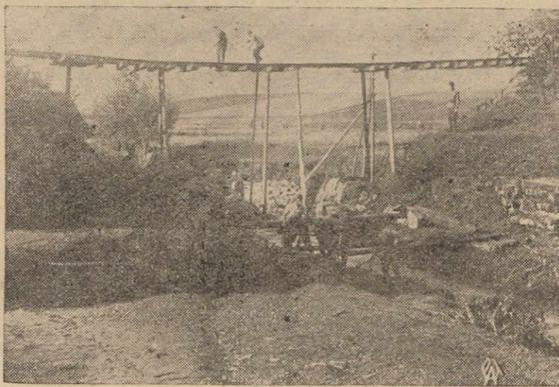
Saperzy przy budowie podpór pod most kolejowy pod stacją kolejową Bogumiłowice, na linii Kraków — Łódź. Most ten długości 130
