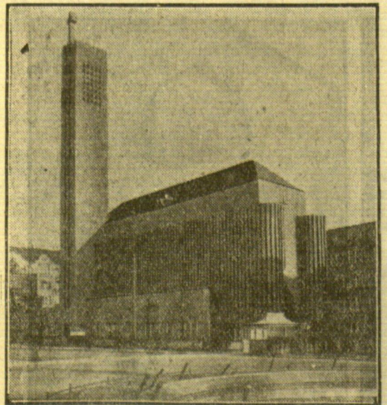
Neuer Kirchenstil
