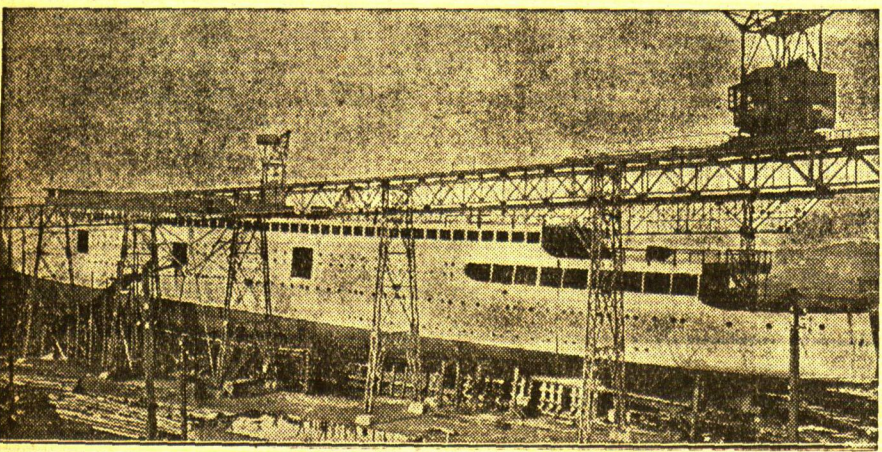
Links: Vor dem Stapellauf des neuen Seebienstampfers „Tannenbera“. Am 16. März wird in Stettin der neue Seebienstampfer „Tannenbera“ vom Stapel laufen, der für den Verkehr zwischen dem Reich und dem Osten bestimmt ist. Das Schiff ist etwa 4000 Tonnen groß und für 2000 Fahrgäste berechnet.
