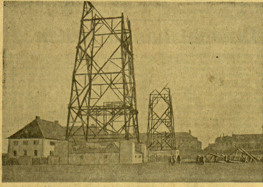
Die Funktürme des Senders München-Stadelheim — eine Holzkonstruktion von 85 Metern Höhe — wurden durch einen Orkan in etwa einem Drittel der Höhe abgebrochen und in einen Trümmerhaufen verwandelt.
