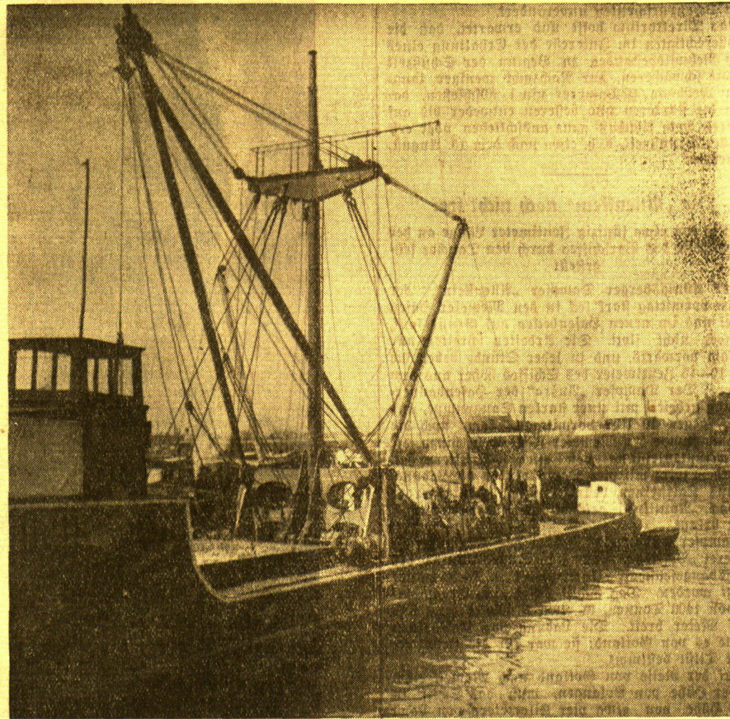
Der im Hafen von Memel auf Grund liegende Dampfer „Allenstein“. Die Aufnahme zeigt die vordere Hälfte des auf Grund liegenden Dampfers. Das Hafenbecken hat hier eine Tiefe von etwa vier Metern, der Tiefgang des Dampfers beträgt etwa dreieinhalb Meter. Das Bild zeigt deutlich, wie tief der Bug des Dampfers sich in das Wasser gesenkt hat; hier stehen sogar die Bullaugen unter Wasser. Der im Hintergrund der Aufnahme sichtbare zweite Dampfer gibt einen guten Vergleichsmassstab ab.
