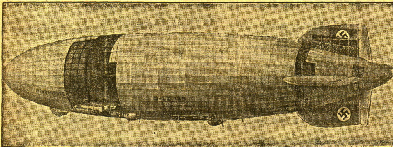
So sieht L 3 129 „Hindenburg“ im Innern aus
