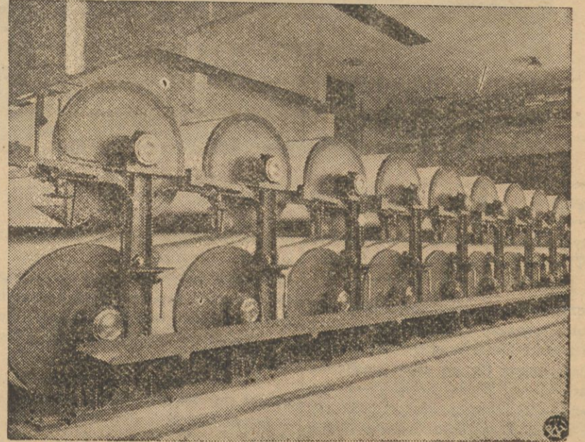
Suszarnia celulozy.
