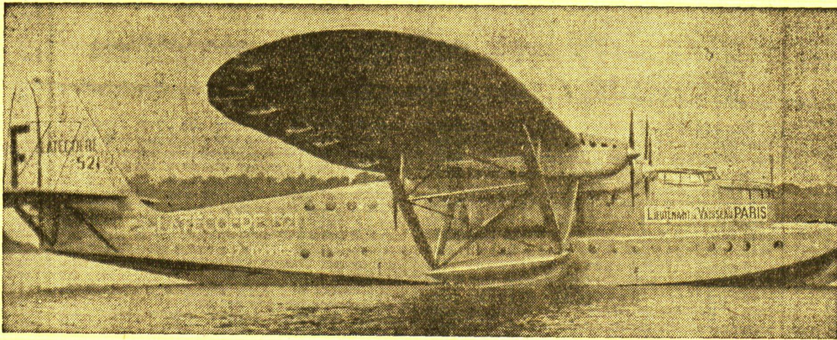
Oben: Das neue französische Großflugboot „Lieutenant de Vaisseau Paris“. Das 37 Tonnen große französische Flugboot „Lieutenant de Vaisseau Paris“ (Schiffsleutnant Paris), hat loeben mit seinen ersten Probeflügen begonnen. Das Flugboot hat eine überragend große Lebnlichkeit mit dem deutschen Flugboot „Do X“ und stellt eine Fortentwicklung dieses Flugboot-Typs dar.
