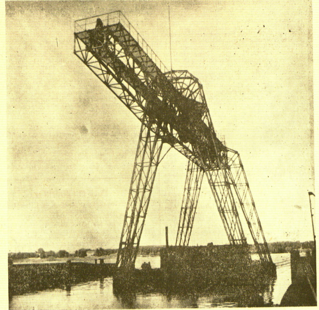
Der 75 000-Kilogramm Schwimmkran
