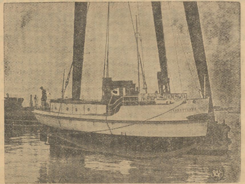
Łódź motorowa przybrzeżna „Samarytanka”, zbudowana w Stoczni Gdynskiej dla Urzędu Morskiego.
