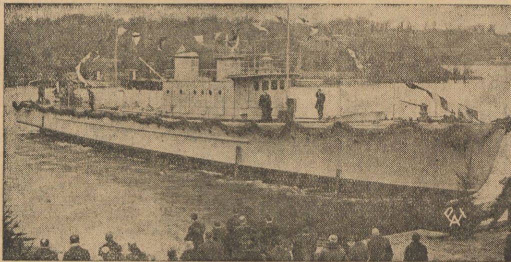
W stoczni modlińskiej Państwowych Zakładów Inżynierii odbyła się w dniu 10 kwietnia b. r. uroczystość spuszczenia na wodę wybudowanego dla Marynarki Wojennej trawlera (okrętu do wyławiania min) „Czajka“. Na zdjęciu — trawler „Czajka“ w chwili po spuszczeniu go na wodę.
