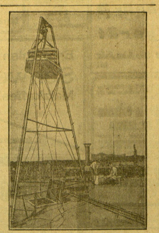
Ein Lautsprecher, der 20 Kilometer überträgt und bei klagerer Wiedergabe eine Lautstärke besitzt, die der eines Orchesters von 2000 Mann entspricht. Dieser Neueste der Radiotechnik, der von einer Berliner Firma gebaut wurde, wird mit einem Strom von 120 Ampere gespeist. Seine Membrane — Aluminiumblech von 1,5 Millimeter Stärke — vibriert Schwingungen bis zu 20 mm Breite aus.
