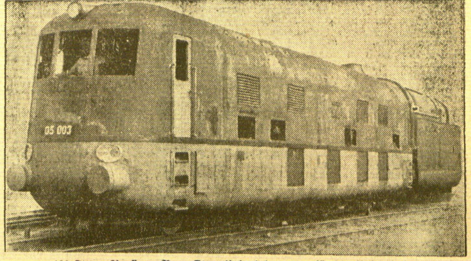
100 Jahre Vorka — Neue Stromlinienlokomotive für die Reichsbahn Zur hundertjährigen Gedenkei, die die Vorka-Werke am 22. Juli begangen, ist gleichzeitig die erste Stromlinienlokomotive, die mit Kohlenstaub betrieben wird und für eine Geschwindigkeit von 175 Stundenkilometer gebaut ist. Für die deutsche Reichsbahn fertig gestellt worden. — Das Bild zeigt den neuen Schienenantrieb. Infolge der automatischen Kohlenstaubfeuerung, die den Heizer von seiner schweren Arbeit weitgehend entlastet, konnte der Führer stand nach vorn verlegt werden, so das man einen ungehinderten Blick über die Strecke hat
