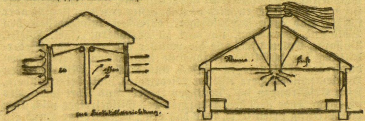
Abb. 3. Luftbewegung im Vakuum-Dachreiter. Abb. 4. Richtige Dachlüftung.
