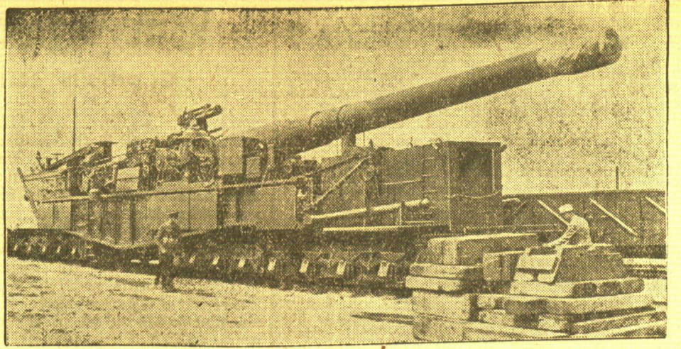
Amerikanisches Riesengeschütz wird an der kalifornischen Küste aufgestellt. Dieses gewaltige 35-Zentimeter-Langrohr-Eisenbahn-Geschütz der amerikanischen Armee, das man acht Jahre lang nicht benutzte, wurde jetzt mit einem Sonderzug von Fort MacArthur nach Saint Clement (Kalifornien) gebracht. Dort soll es wieder eingeschossen werden. Das Geschütz hat eine Reichweite von 32 Kilometer.
