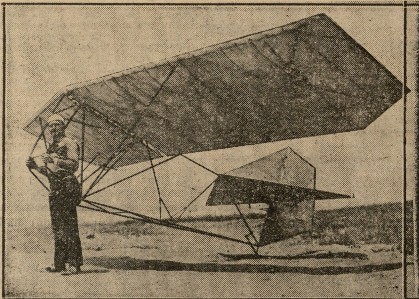
Po czteroletnich pracach i próbach Amerykanin Bob Morse wynalazł szybowiec, wprawiany w ruch bez pomocy katapulty, a osiągający szybkość 35 km na godz. Kierunek i wysokość lotu zależna jest w tym aparacie od ruchów ciała pilota.
