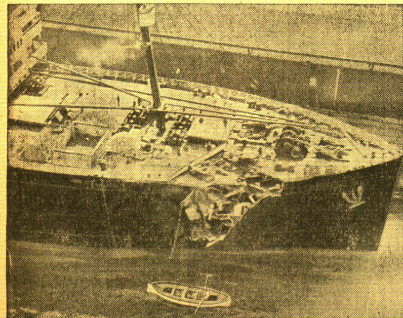
Schiffszusammenstoß im Nebel der Irischen See Etwa sechs Meilen vor Liverpool stieß im dichten Nebel der Frachtdampfer „Napier Star“ mit dem Passagierdampfer „Laurentic“ zusammen. Dabei wurde die Bordwand der „Laurentic“ bis zum Laderraum aufgerissen. Man sieht auf unserem Bild das havarierte Schiff nach dem Einschleppen in den Hafen.
